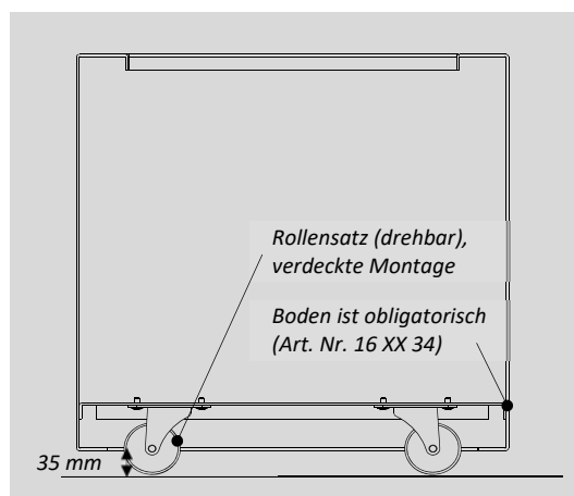
Beispiel Rollensatz mit Pflanzgefäß als Schemazeichnung...
