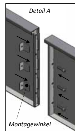
Eckkombination von Pflanzgefäßen. Länge 4,0 m, Höhe 0,5 m bzw. 0,25 m
