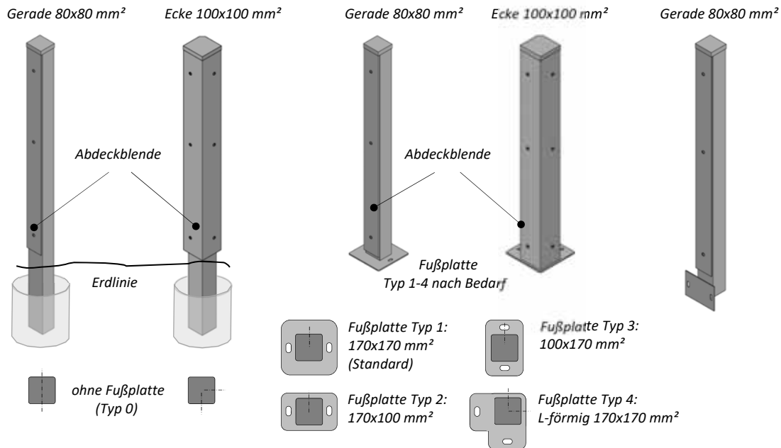
Zaunpfosten BOSTON zum Einbetonieren
