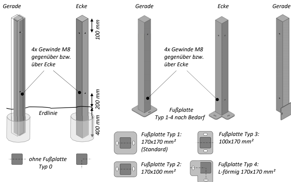
Befestigung Zaunpfosten MIAMI zum Einbetonieren
