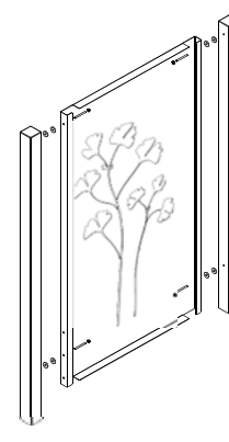
Montage VISTA zwischen Zaunpfosten
