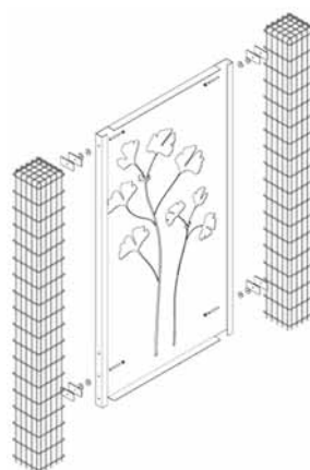
Montage VISTA zwischen Gabionkörben
