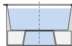
Badefass AQUA LUND mit integrierter 360°-Sitzbank vorbereitet für externe Heizung
