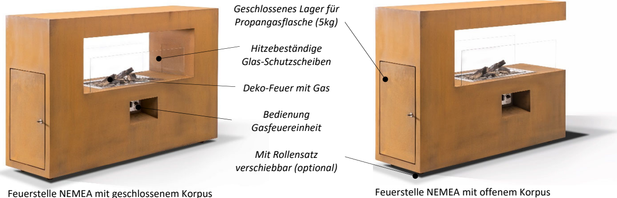
Feuerstelle NEMEA mit geschlossenem Korpus
