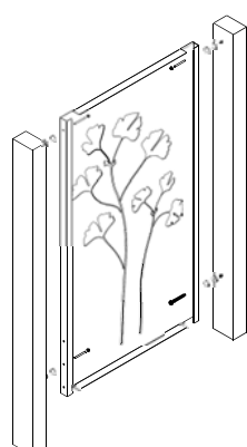
Montage VISTA zwischen Holzpalisaden oder Holzbalken
