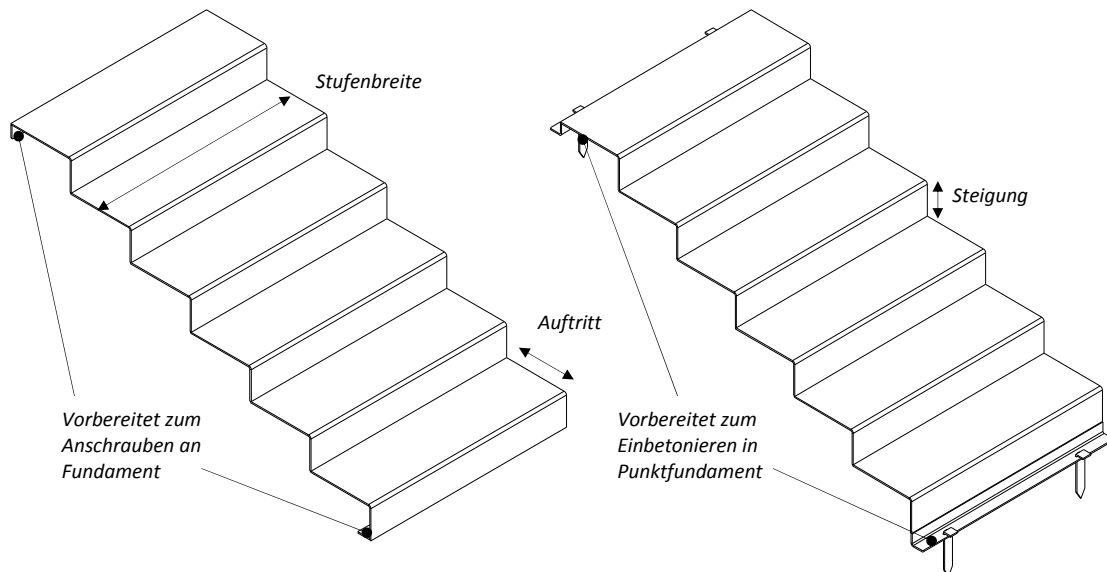
Variante A: Massiv-Treppe zum Anschrauben
