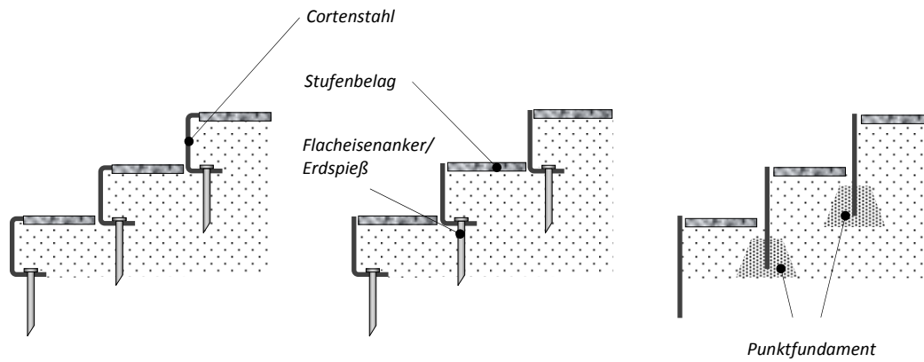
Treppenstufen Typ C-Form
