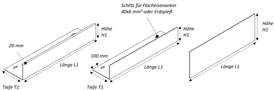
Treppenstufe Typ C-Form
