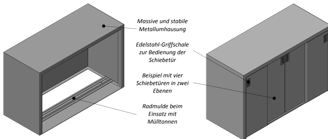
Mülltonnen- und Fahrradbox ohne Schiebetüren
